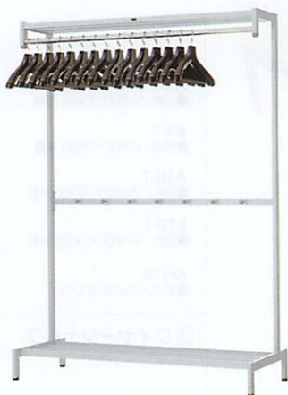
CH-3 ●規格/W900×D480×H1650
